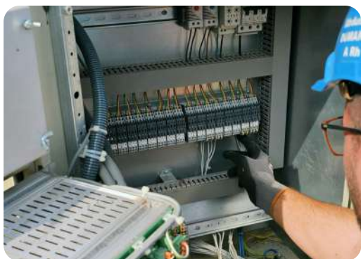
Cableado Eléctrico
